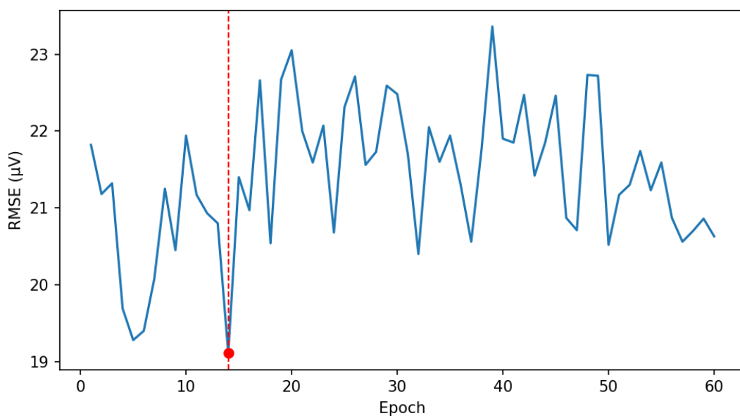
FIGURE 12 – S004 — Évolution du RMSE par epoch (ART vs ICLabel, checkpoints LOSO).
