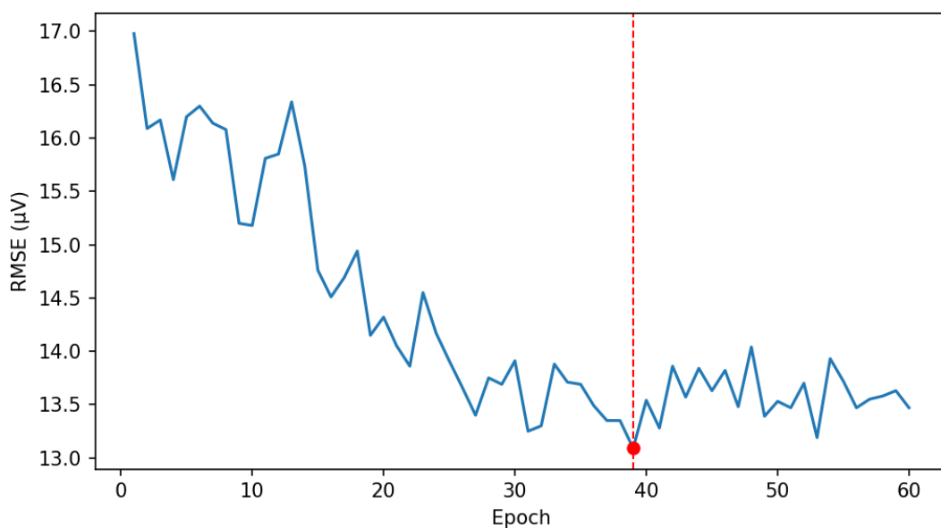
FIGURE 15 – S005 — Évolution du RMSE par epoch (ART vs ICLabel, checkpoints LOSO).
