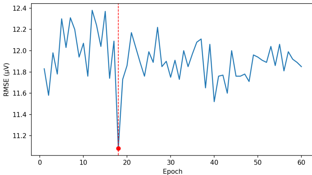
FIGURE 6 – S002 — Évolution du RMSE par epoch (ART vs ICLabel, checkpoints LOSO).
